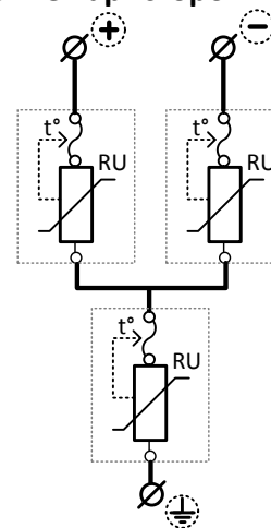
Рисунок 2. Электрическая схема УЗИП Комменж УЗФЭС-3 150/10У
