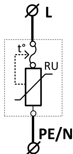
Рисунок 2. Функциональная схема подключения к электроустановке
