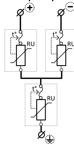
Рисунок 2. Электрическая схема УЗИП Комменж УЗФЭС-3 800/10У
