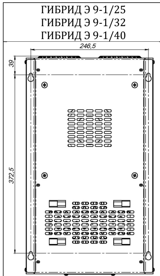
Рисунок 4. Установочные размеры стабилизаторов
