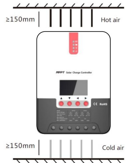
Рисунок 2-1. Установка и рассеивание тепла
