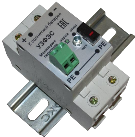
Рисунок 1. Внешний вид УЗИП Комменж УЗФЭС-3 600/10У
