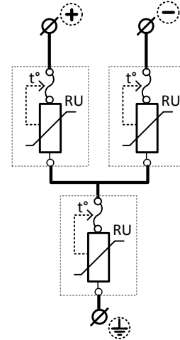
Рисунок 2. Электрическая схема УЗИП Комменж УЗФЭС-3 600/10У
