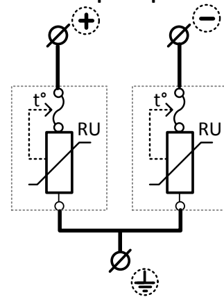
Рисунок 2. Электрическая схема УЗИП Комменж УЗФЭС-2 75/40V
