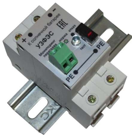
Рисунок 1. Внешний вид УЗИП Комменж УЗФЭС-2 75/40V
