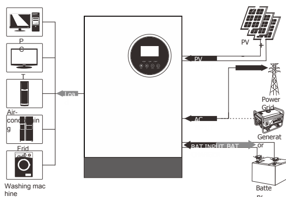
Рисунок 1 Гибридный солнечный инвертор
