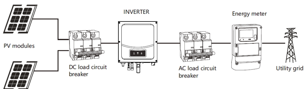
Рисунок 5 Схема подключения инвертора в электрохозяйство без функции ограничения отдачи электроэнергии в сеть
