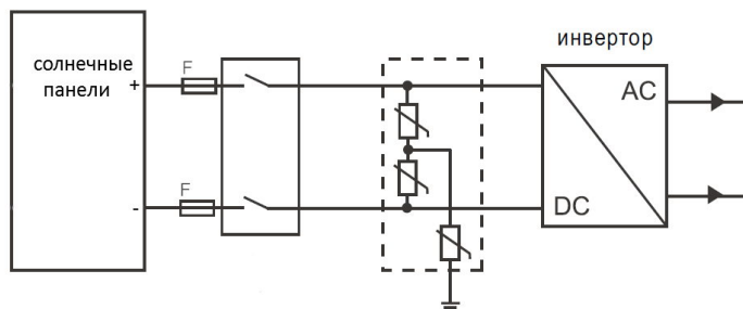
Рисунок 13 Принципиальная схема установки предохранителей и УЗИП в линию постоянного тока
