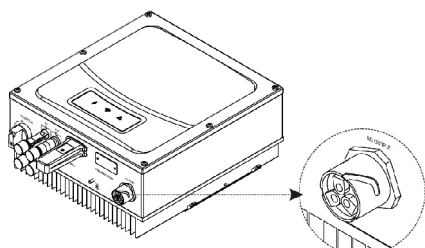
Рисунок 8 Силовой разъём AC на корпусе инвертора
