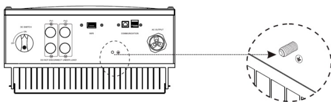
Рисунок 9 Расположение клеммы заземления
