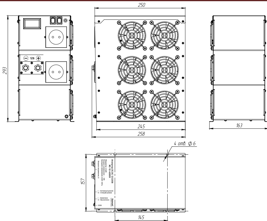
Рисунок 1 – Внешний вид инвертора
