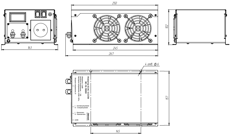
ИС-12/24-1500У
