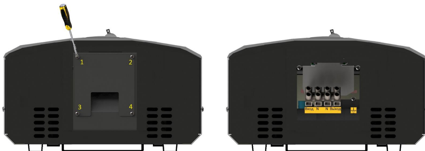
Рисунок 11. Схема снятия защитной крышки снизу корпуса стабилизатора
