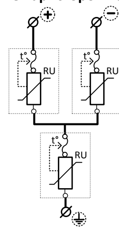
Рисунок 2. Электрическая схема УЗИП Комменж УЗФЭС-2 800/40У
