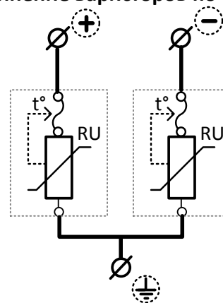
Рисунок 2. Электрическая схема УЗИП Комменж УЗФЭС-2 150/80V
