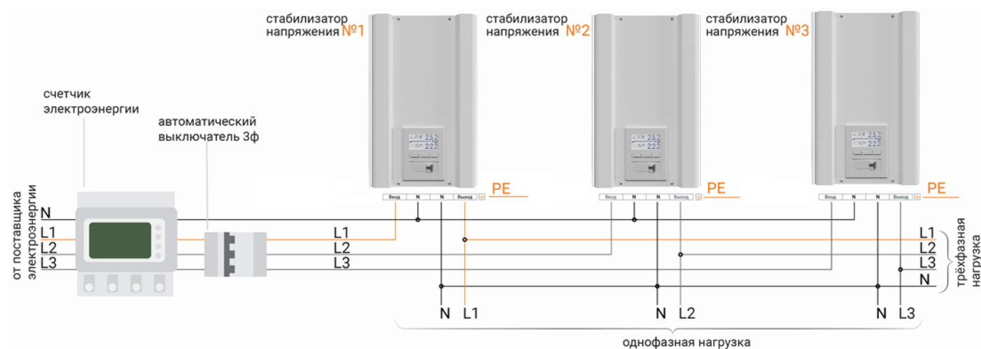
Рисунок 7. Схема подключения стабилизатора к трёхфазной сети
