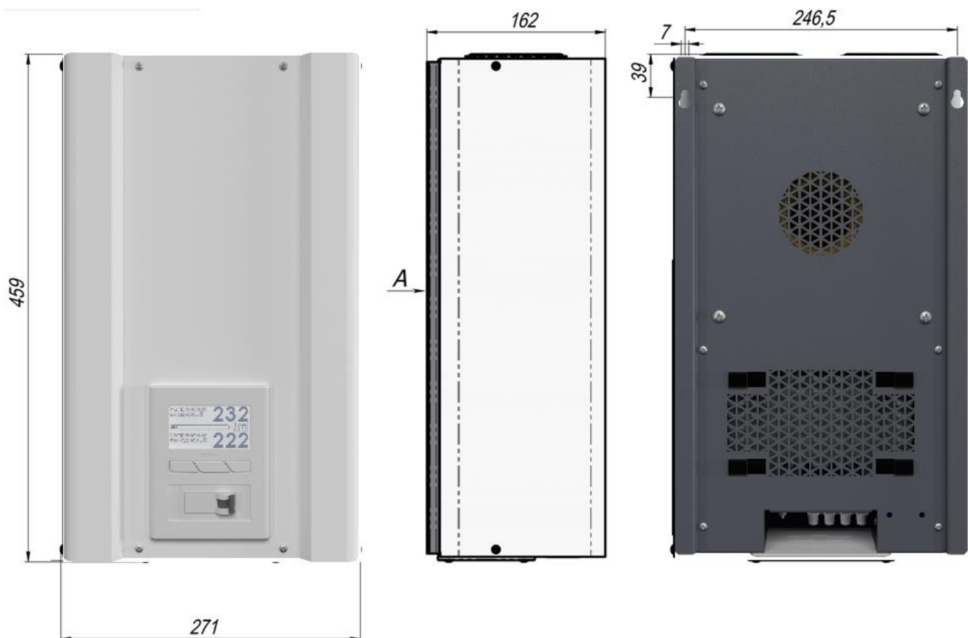
Рисунок 4. Габаритные и установочные размеры стабилизаторов АМПЕР на 25, 32, 40А
