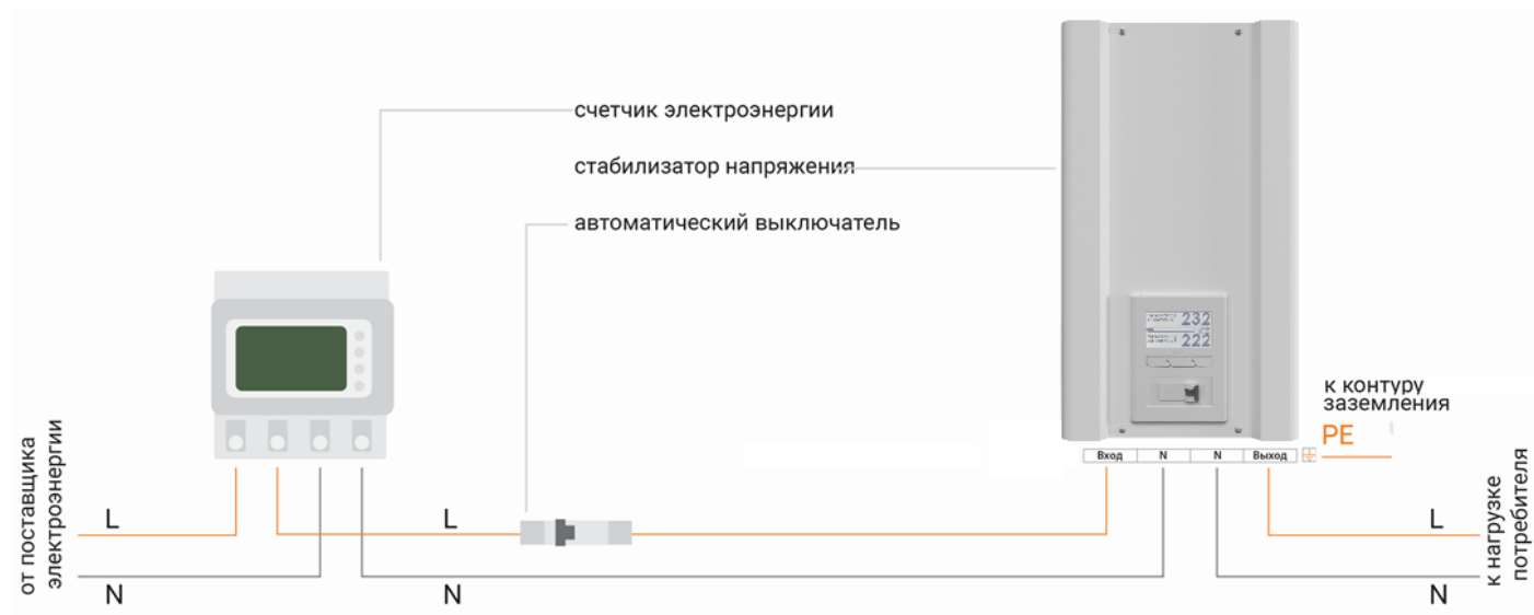
Рисунок 6. Схема подключения стабилизатора к однофазной сети
