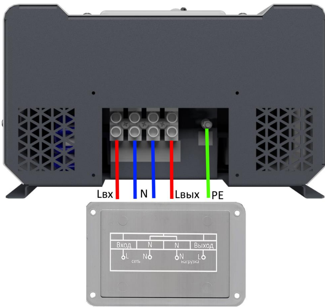
Рисунок 8. Схема подключения стабилизатора
