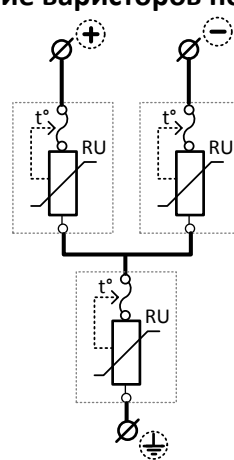
Рисунок 2. Электрическая схема УЗИП Комменж УЗФЭС-2 150/40У
