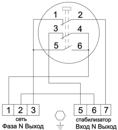
Рисунок 1 – Схема подключения байпаса однофазного ручного
