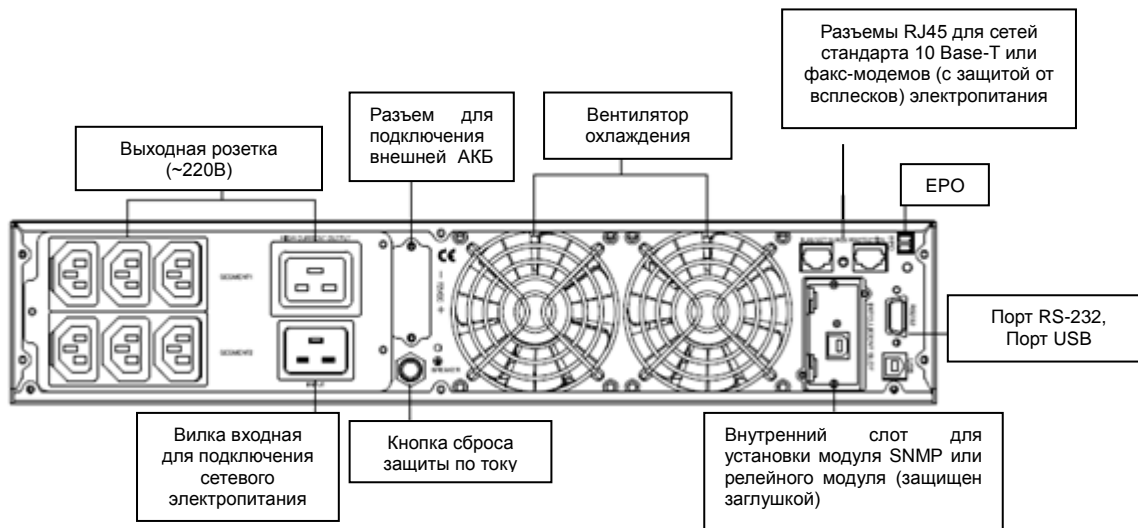
Рис. 4 Вид задней панели 3КВА
