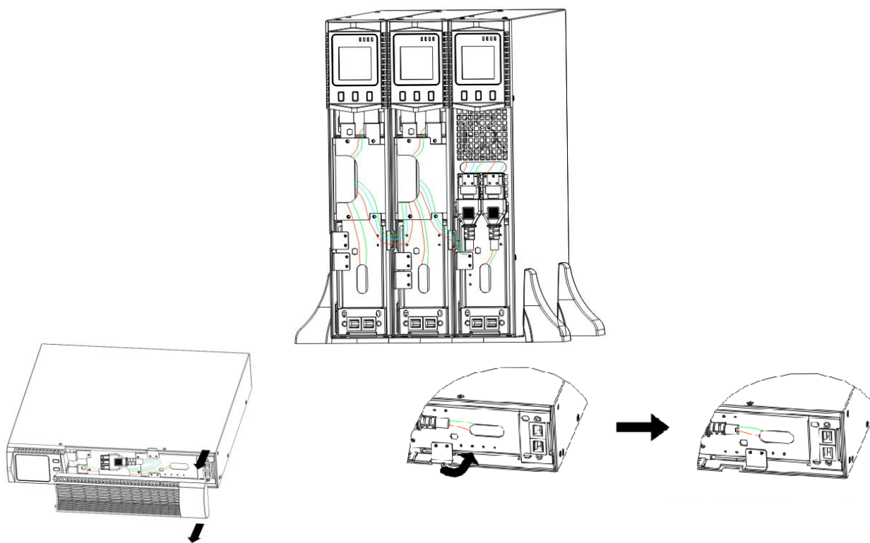
Рис. 8 Подключение дополнительного батарейного кабинета
