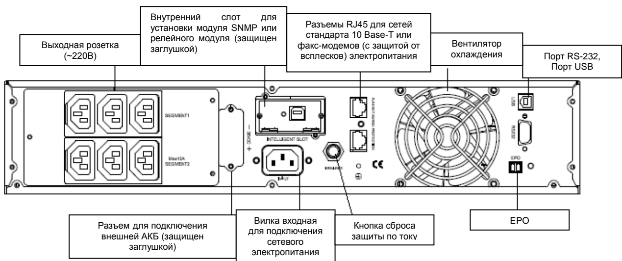
Рис. 3 Вид задней панели 1кВА
