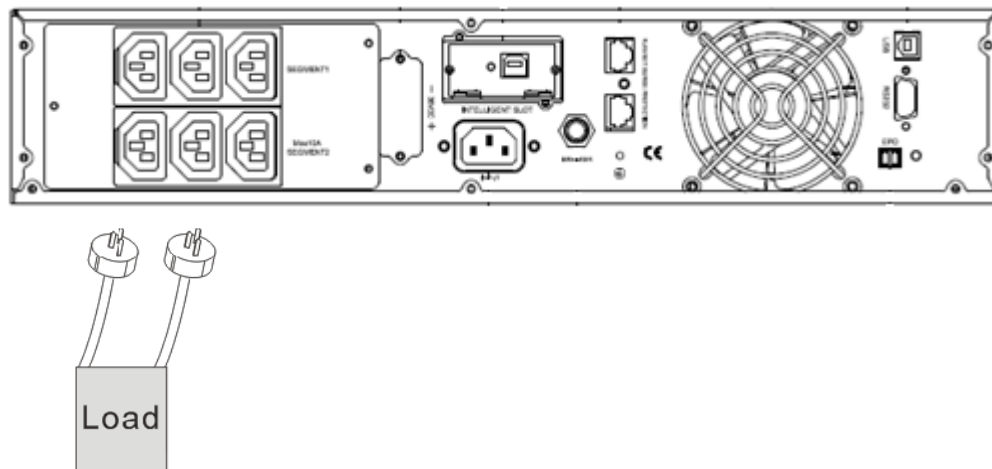
Рис. 7 Подключение нагрузки
