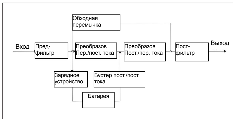
Рис. 5 Принципиальная схема ИБП
