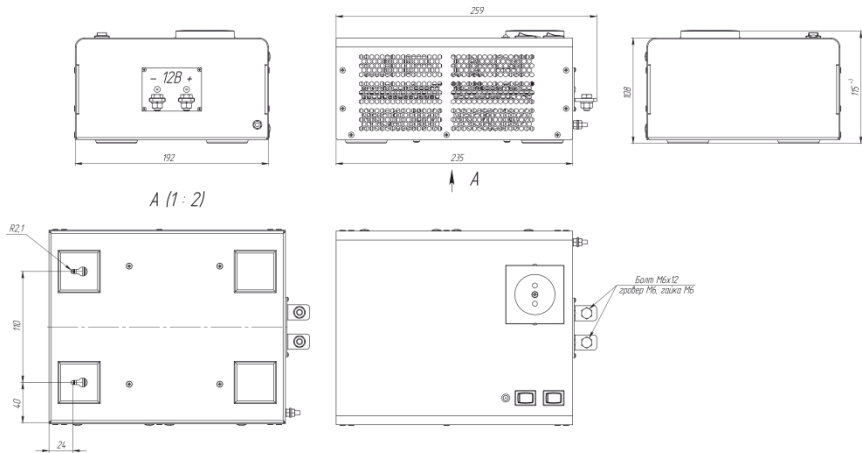
Рисунок 1. Внешний вид СибВатт 1712
