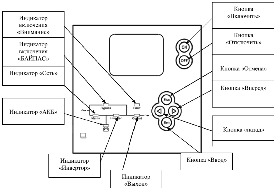
Рисунок 3 - Информационная передняя панель
