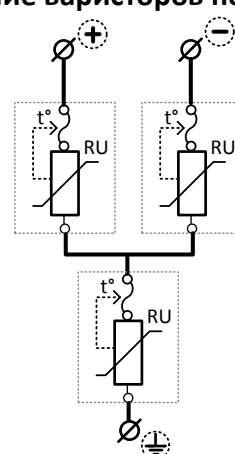
Рисунок 2. Электрическая схема УЗИП Комменж УЗФЭС-2 600/40У
