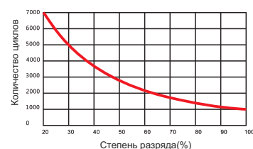
Зависимость циклов от глубины разряда
