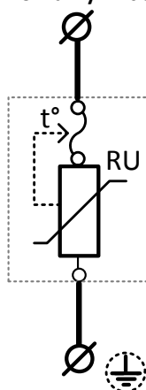
Рисунок 2. Электрическая схема добавочного УЗИП Комменж УЗФЭС-Д 75/40
