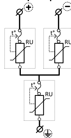
Рисунок 2. Электрическая схема УЗИП Комменж УЗФЭС-2 150/15У
