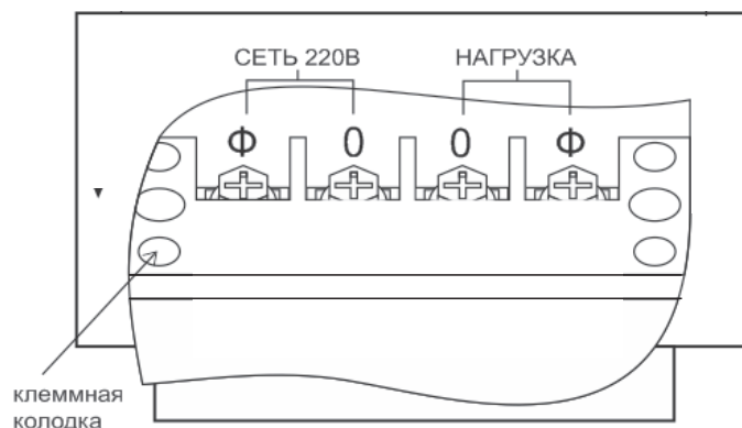
Рисунок 3 – Схема подключения к клеммной колодке
