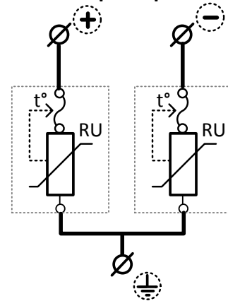
Рисунок 2. Электрическая схема УЗИП Комменж УЗФЭС-2 600/40V
