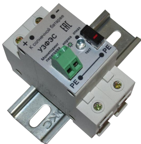
Рисунок 1. Внешний вид УЗИП Комменж УЗФЭС-2 600/15У
