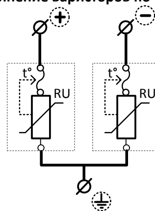
Рисунок 2. Электрическая схема УЗИП Комменж УЗФЭС-2 300/40V
